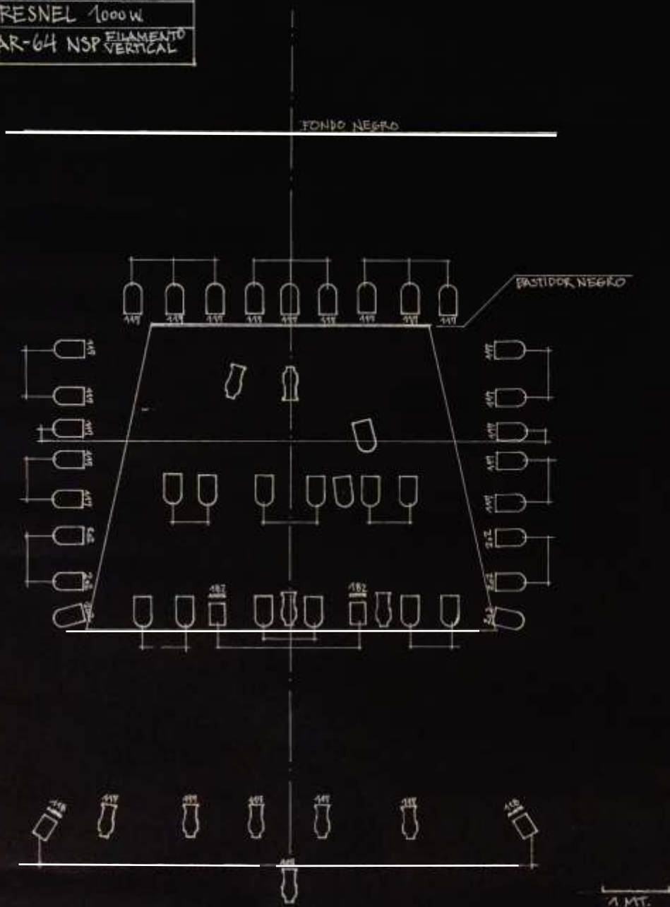
• PLANTA DE ILUMINACION DE "NO 7" • 2015 • ESCALA 1:50 •
